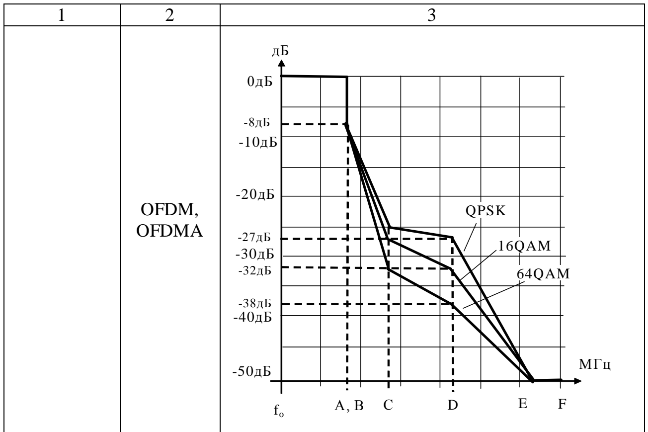
Координаты точек перегиба масок спектра
